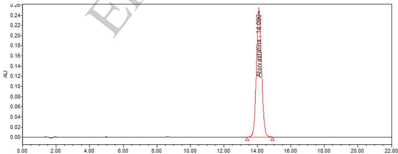
Figura 1. Cromatograma guía obtenido de la solución estándar.
