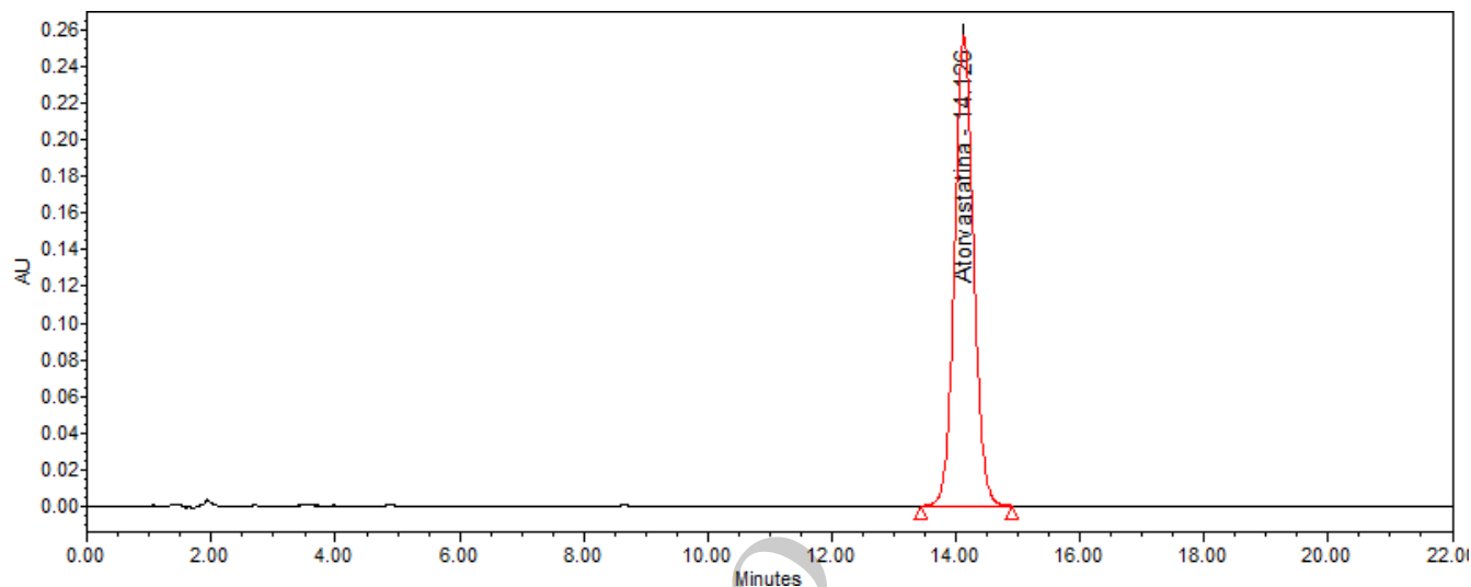
Figura 2. Cromatograma guía obtenido de la solución muestra
