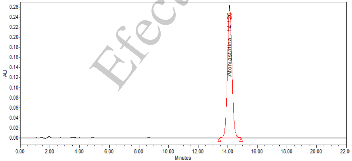
Figura 8. Cromatograma Guía obtenido de la solución Muestra
